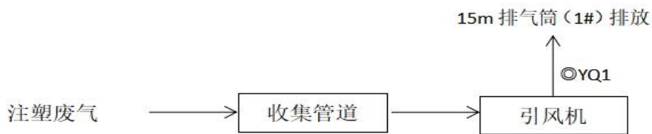
图 3-2 废气处理工艺
