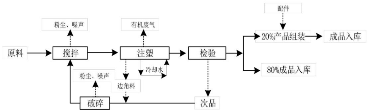
图 2-2 项目生产工艺流程图
